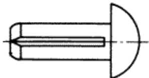
Halbrundkerbnagel DIN 1476 bzw. ISO 8746 Form A mit Fase (Standard)
